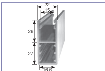
Profil za rolete
