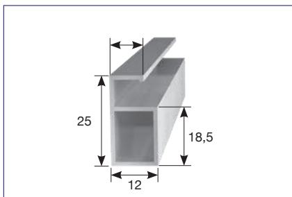
Profil za komarnik
