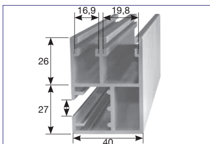
Profil za rolete
